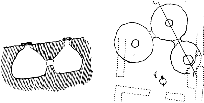
شكل 4 - مطامير قلعة بني حماد ، تصميم ومقطع ( عن لوسيان قولفين )
